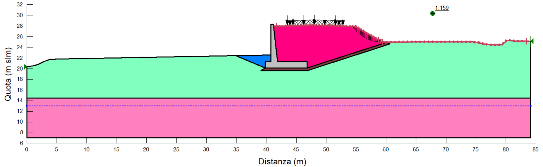
Figura 10.3: Rilevato delimitato da muro di sostegno, sez. 0+500 - Analisi di stabilità globale in campo statico DA1C2 – Parametri non drenati
