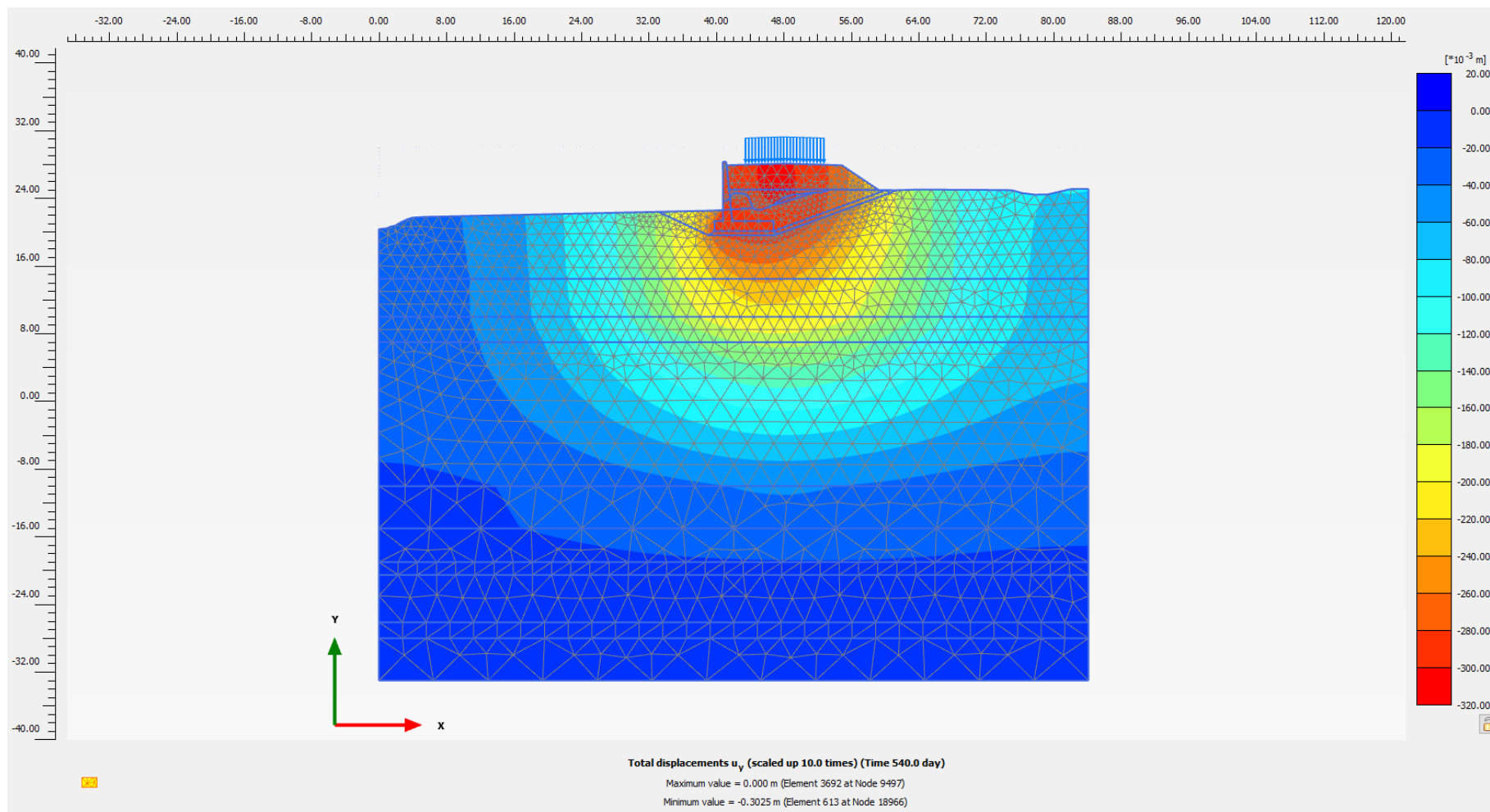
Figura 10.8: Rilevato sez. 0+500 – Spostamenti verticali termine costruzione
