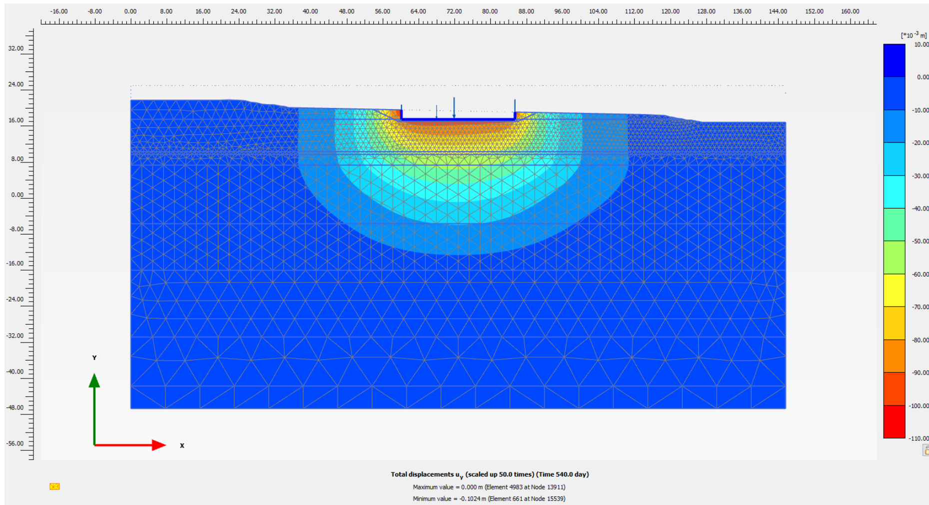
Figura 11.6: Scatolare sez. 1+775 – Spostamenti verticali termine costruzione
