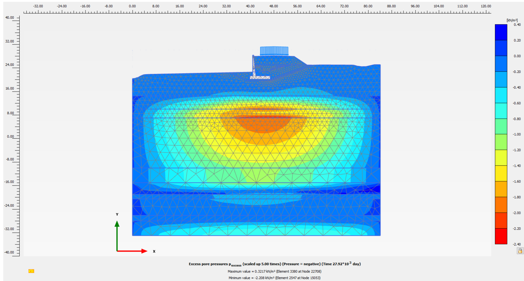
Figura 10.11: Rilevato sez. 0+500 – Sovrappressioni interstiziali \Delta u lungo termine
