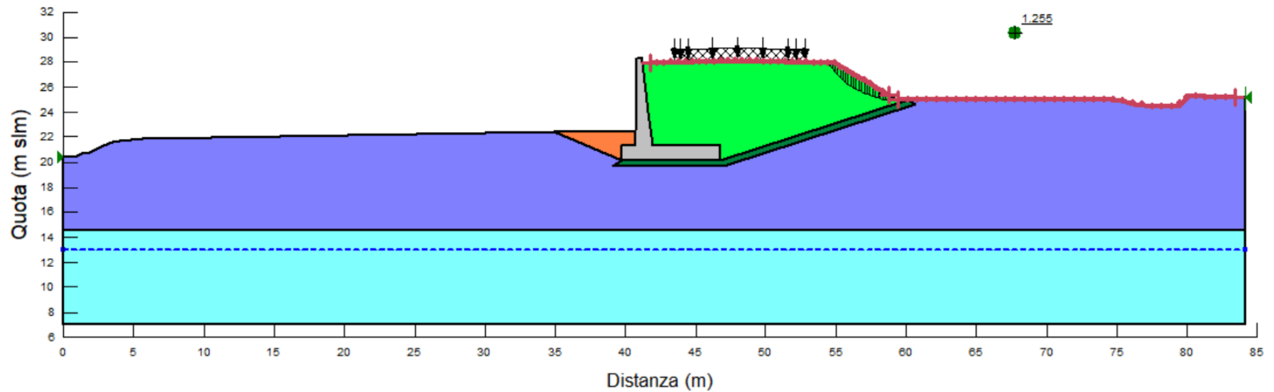
Figura 10.4: Rilevato delimitato da muro di sostegno, sez. 0+500 - Analisi di stabilità globale in campo sismico
