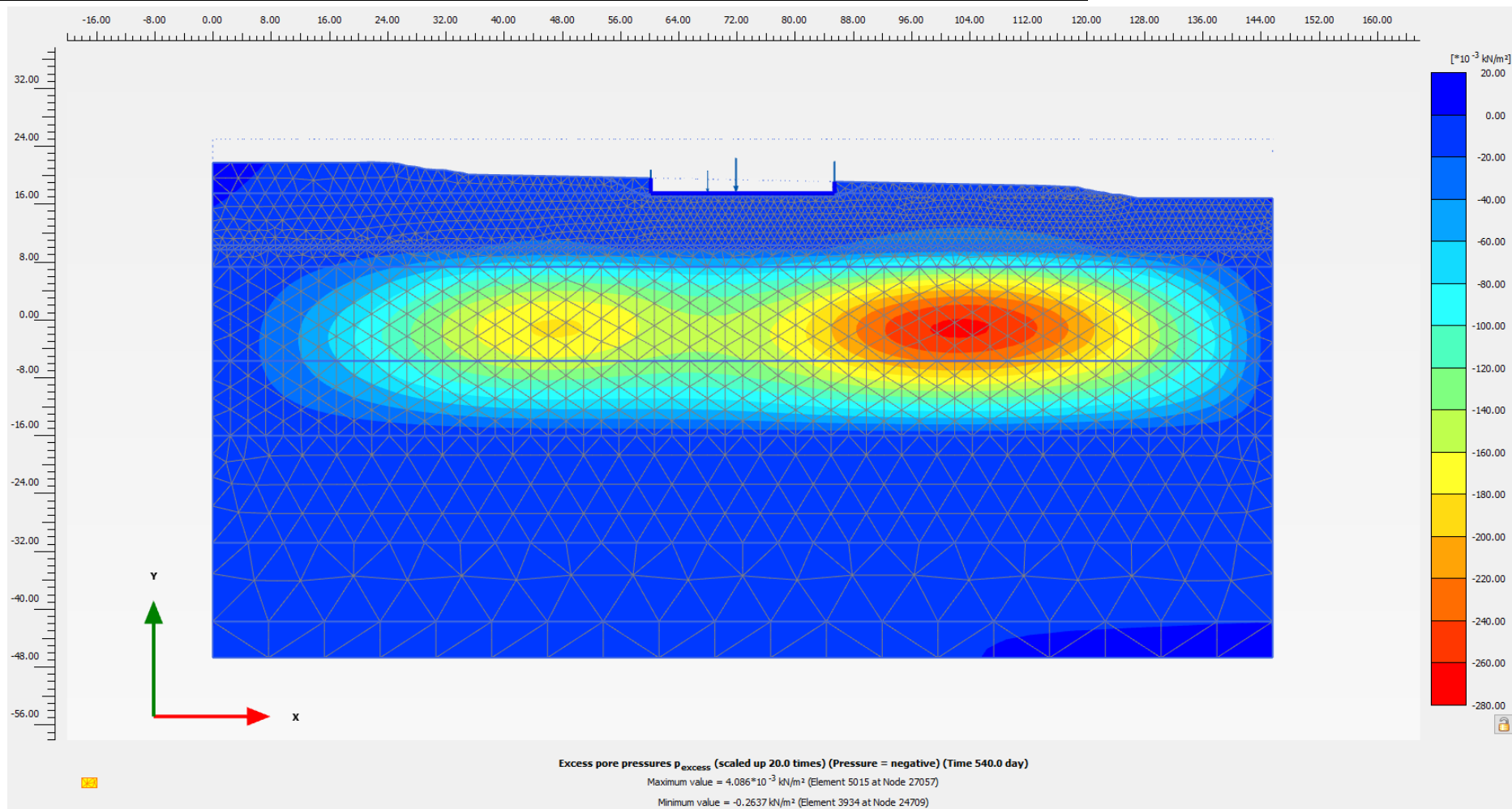
Figura 11.8: Scatolare sez. 1+775 – Sovrappressioni interstiziali \Delta u termine costruzione
