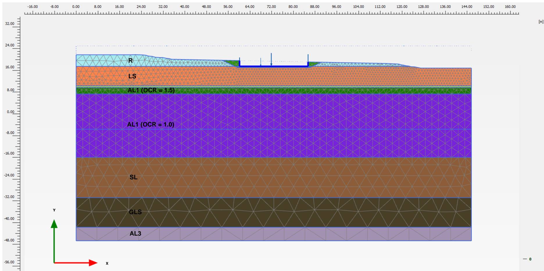
Figura 11.3: Modello Scatolare Stazione Tor di Quinto, sez. 1+775
