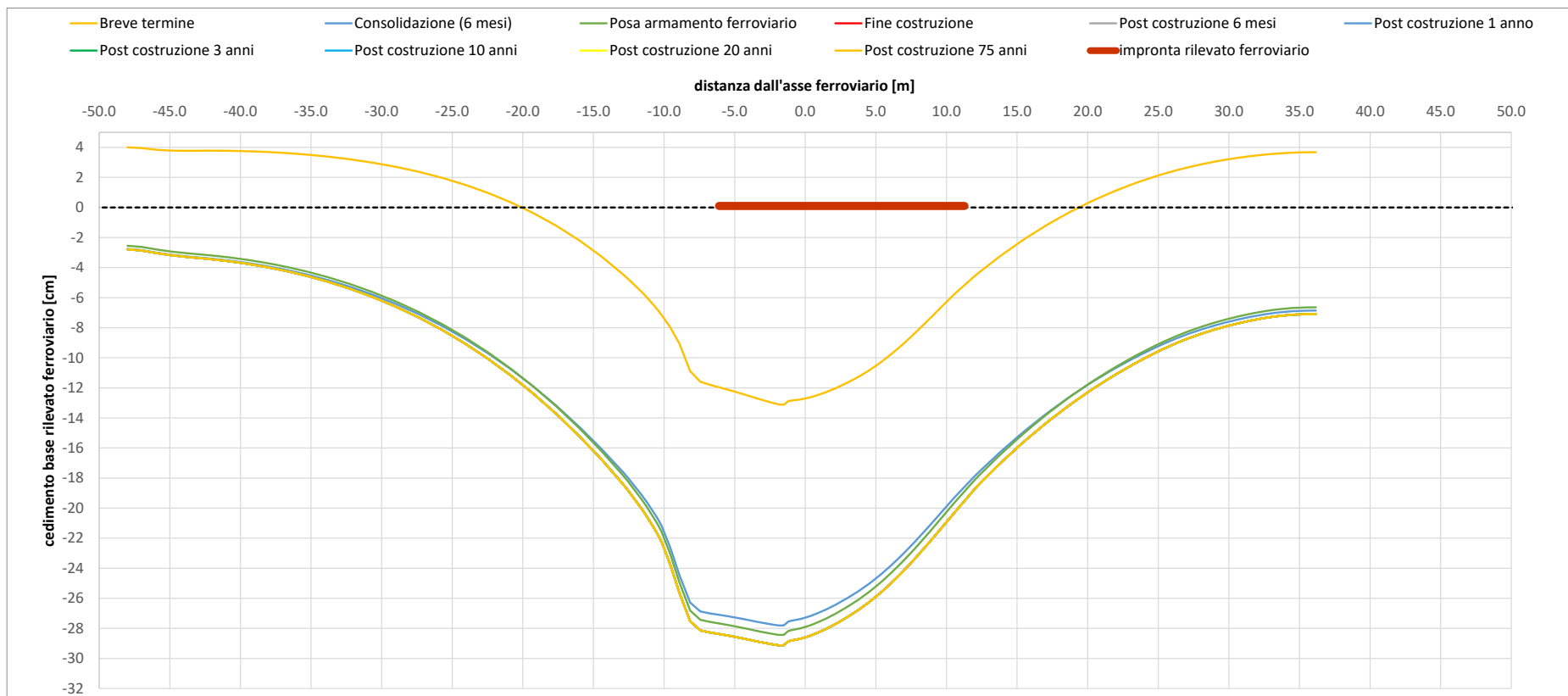
Figura 10.7: Rilevato sez. 0+500 – Spostamenti verticali in corrispondenza della base del rilevato ferroviario
