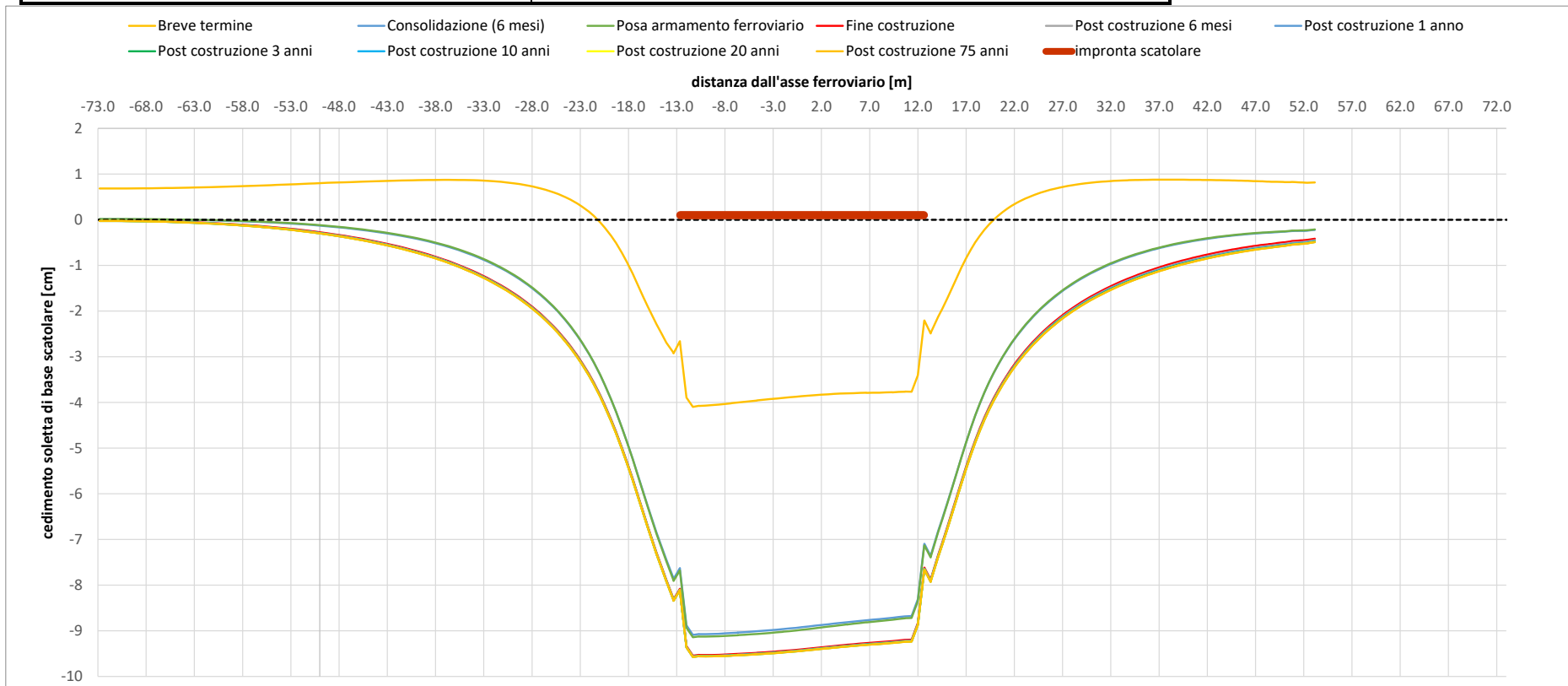
Figura 11.5: Scatolare sez. 1+775 – Spostamenti verticali in corrispondenza della soletta di base dello scatolare
