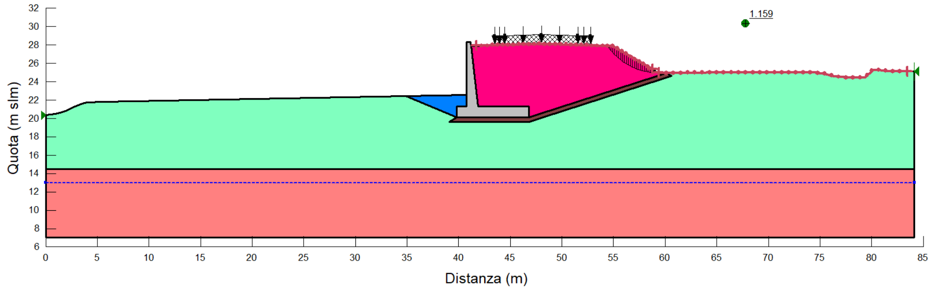
Figura 10.2: Rilevato delimitato da muro di sostegno, sez. 0+500 - Analisi di stabilità globale in campo statico DA1C2 – Parametri drenati
