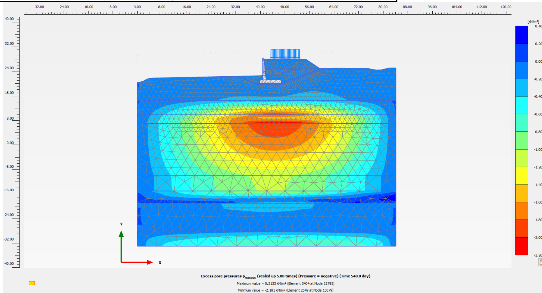
Figura 10.10: Rilevato sez. 0+500 – Sovrappressioni interstiziali \Delta u termine costruzione
