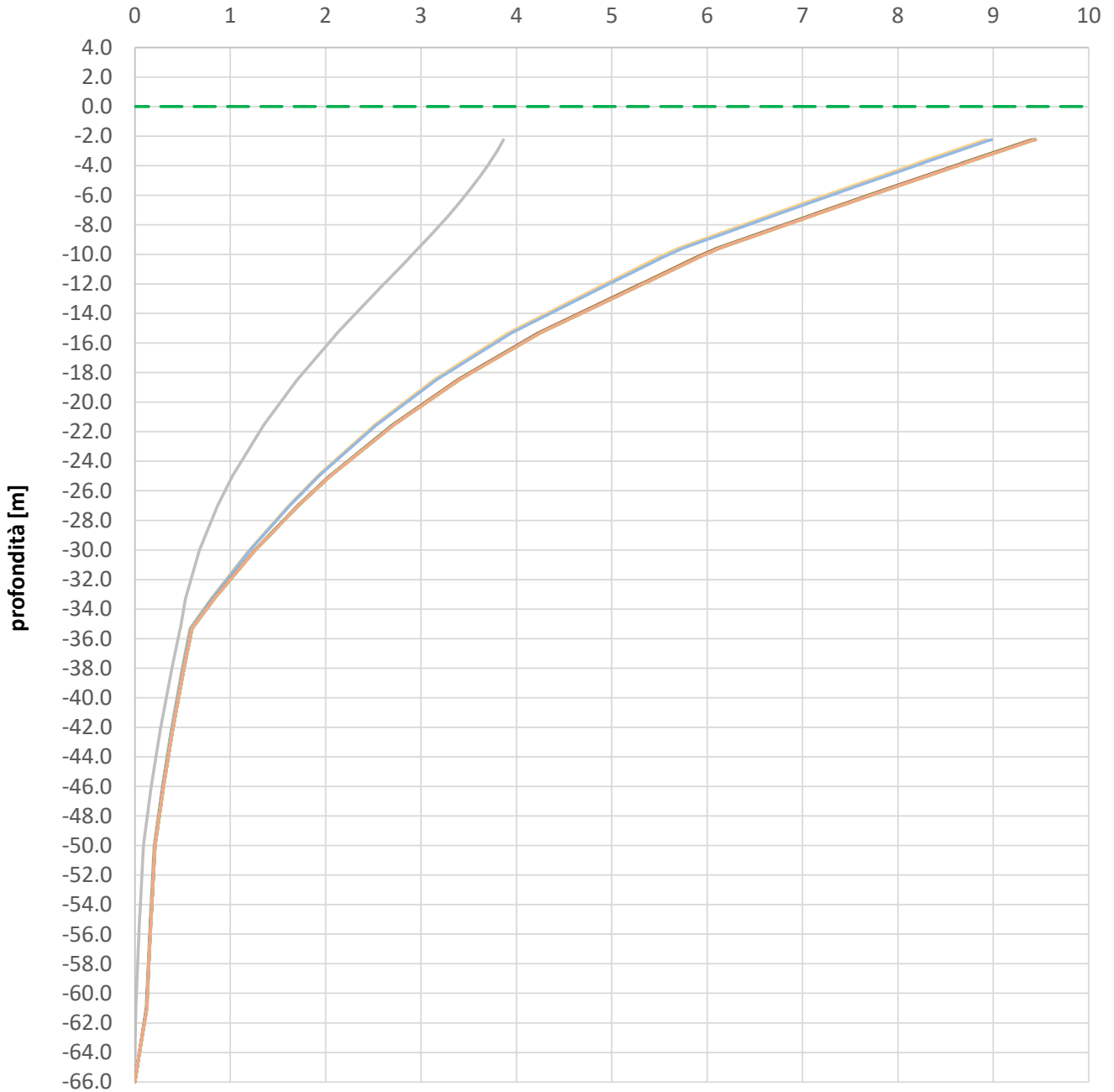
Figura 11.4: Scatolare sez. 1+775 – Spostamenti verticali in corrispondenza del centro della soletta di base dello scatolare
