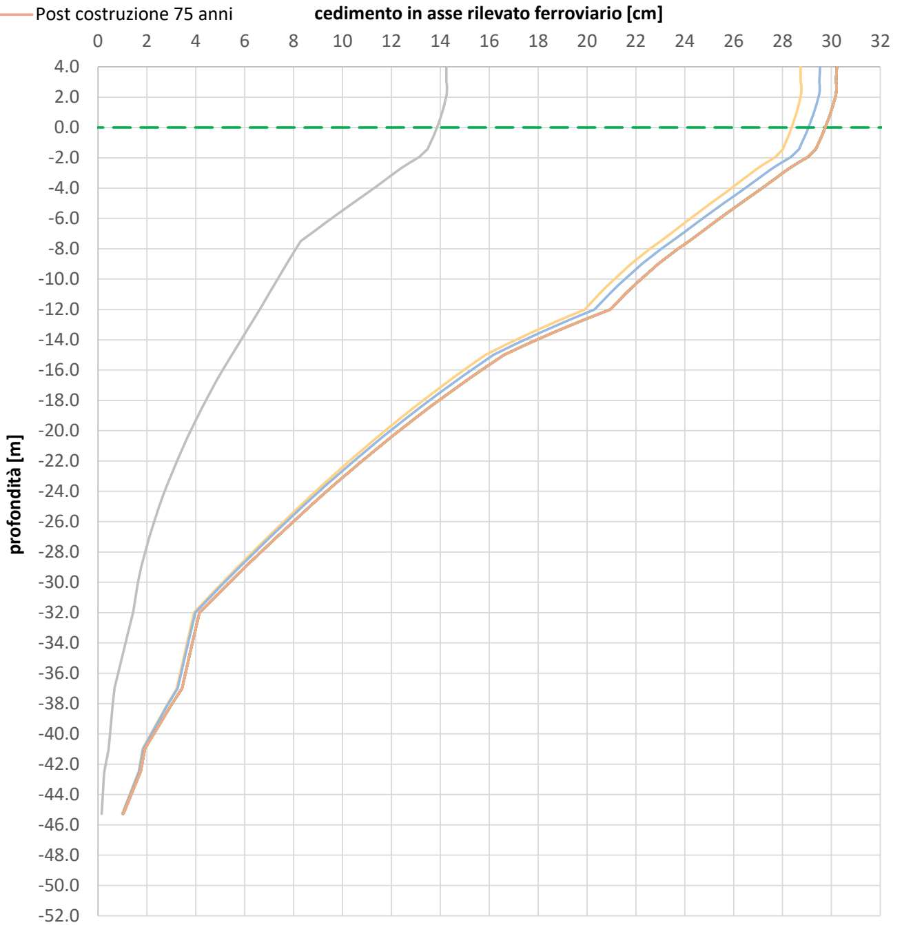
Figura 10.6: Rilevato sez. 0+500 – Spostamenti verticali in corrispondenza del centro del rilevato
