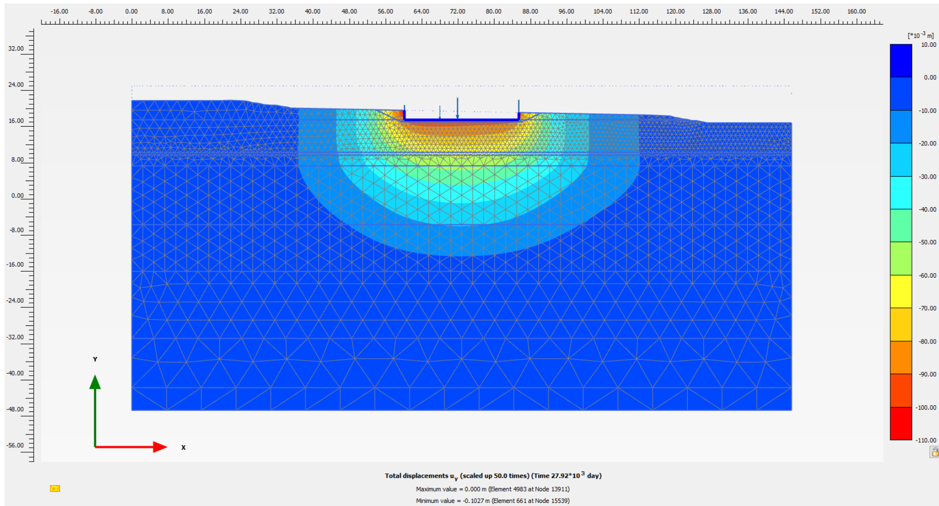
Figura 11.7: Scatolare sez. 1+775 – Spostamenti verticali lungo termine
