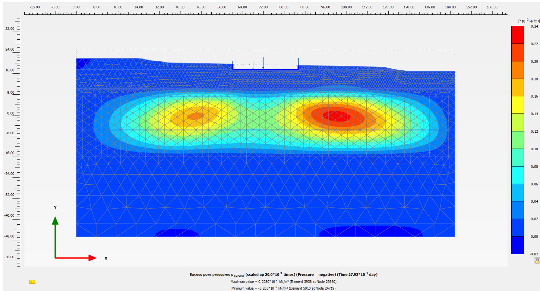
Figura 11.9: Scatolare sez. 1+775 – Sovrappressioni interstiziali \Delta u lungo termine
