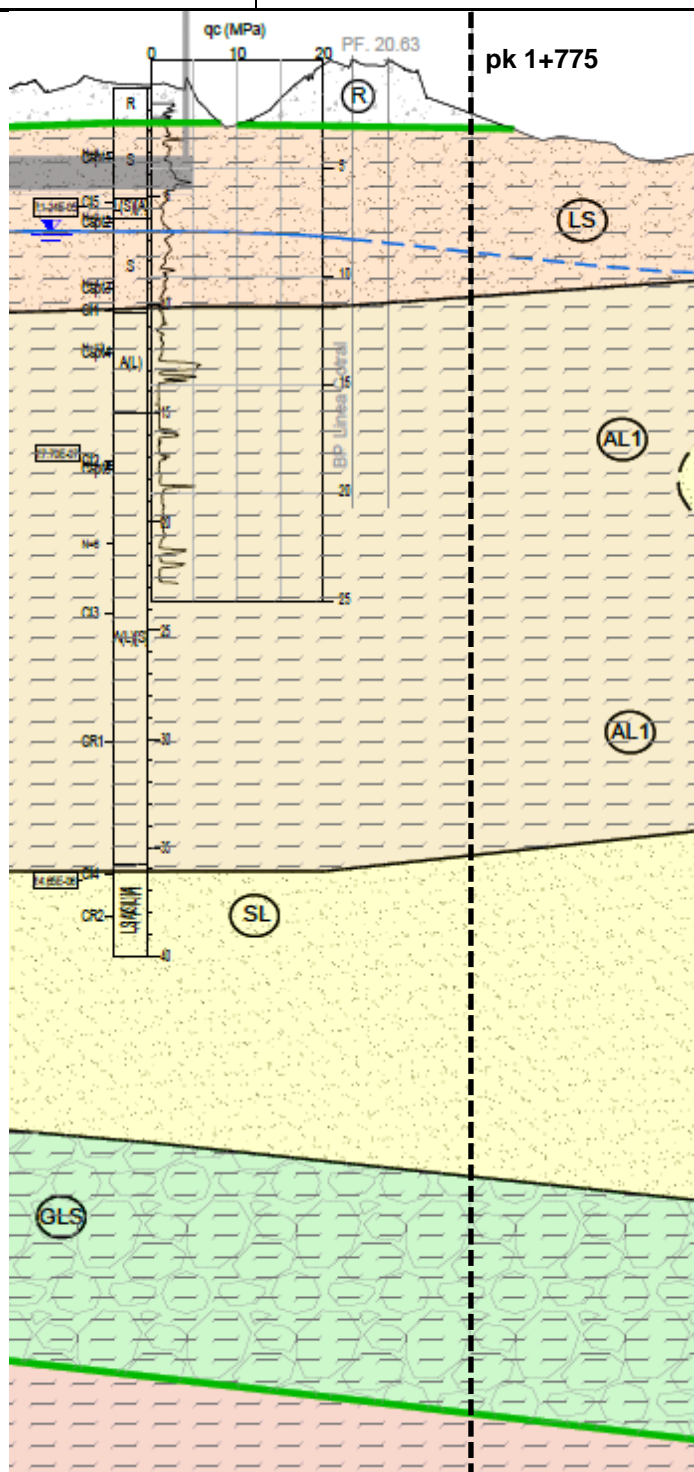
Figura 11.1: Stralcio del Profilo geotecnico in corrispondenza della sezione al km 1+775
