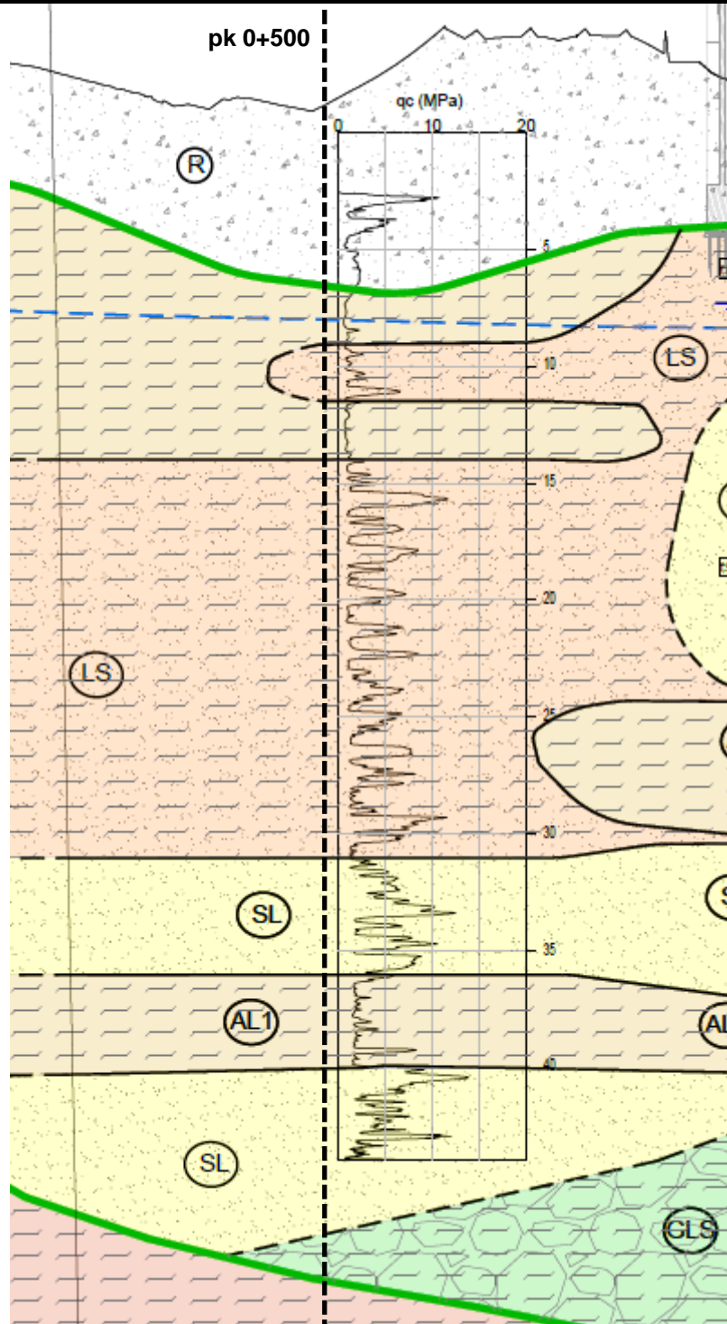
Figura 10.1: Stralcio del Profilo geotecnico in corrispondenza della sezione al km 0+500
