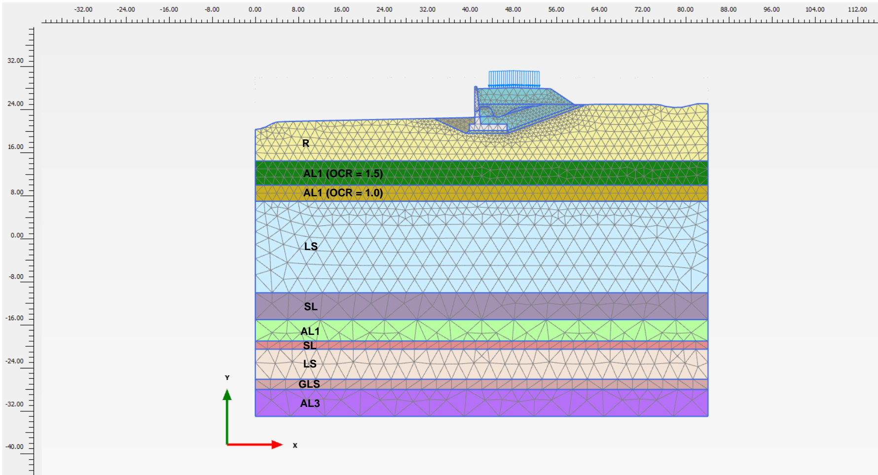
Figura 10.5: Modello rilevato Sez. 0+500
