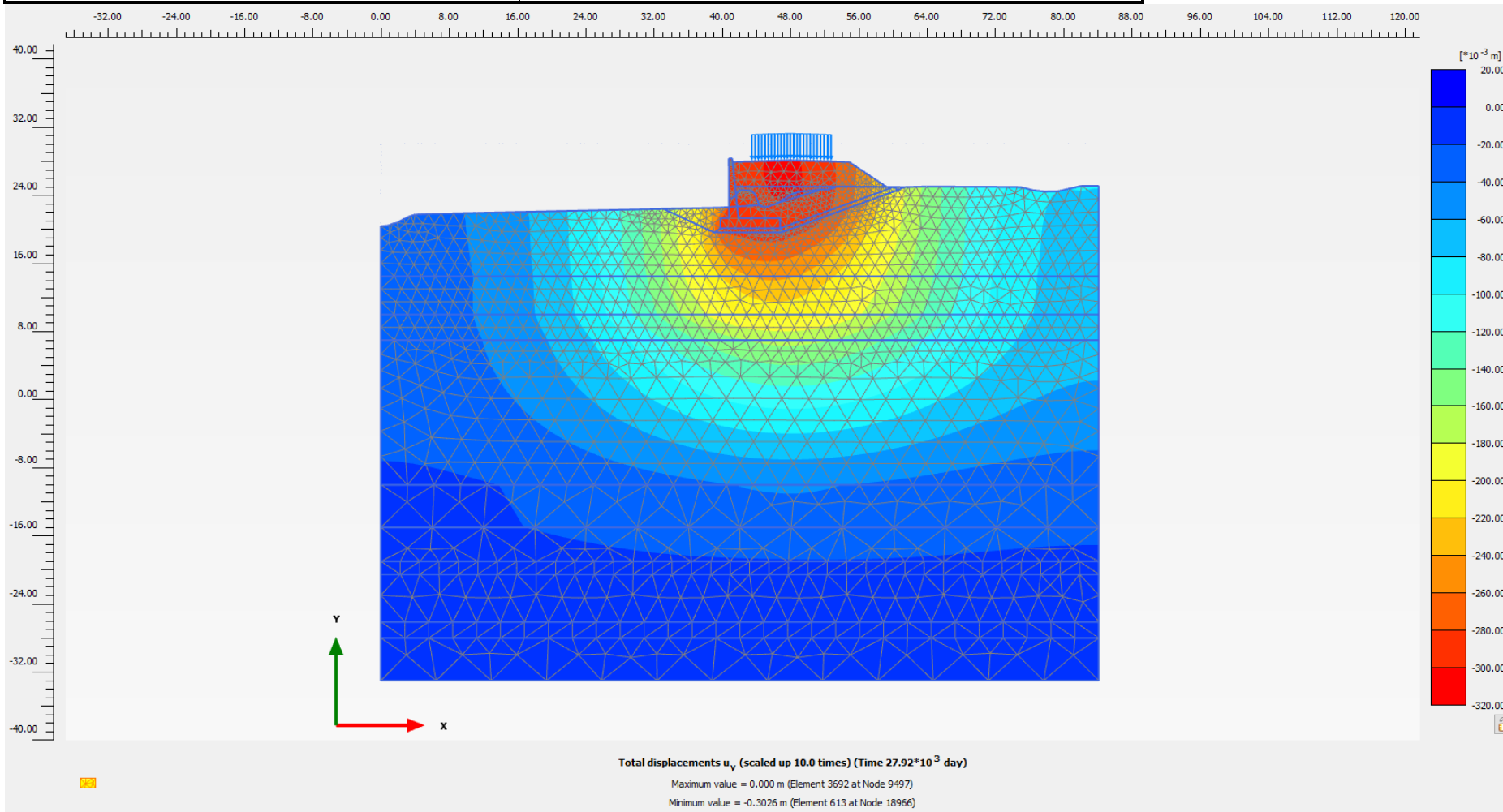
Figura 10.9: Rilevato sez. 0+500 – Spostamenti verticali lungo termine
