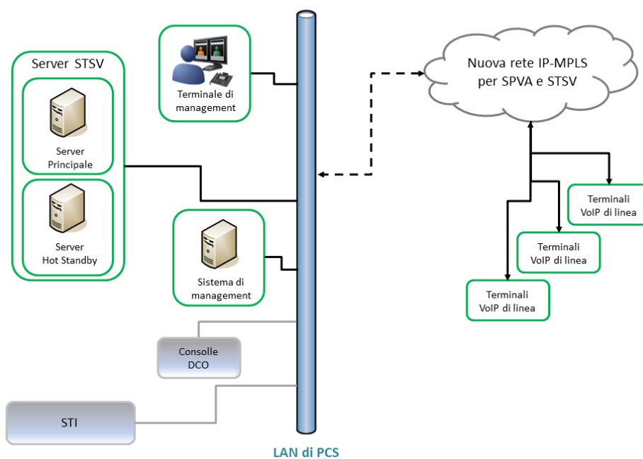
Figura 3: Architettura Sistema Telefonia Selettiva STSV
