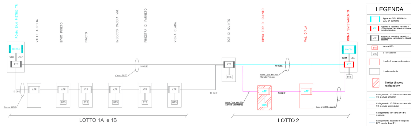
Figura 2: Architettura della rete di trasporto MPLS-TP
