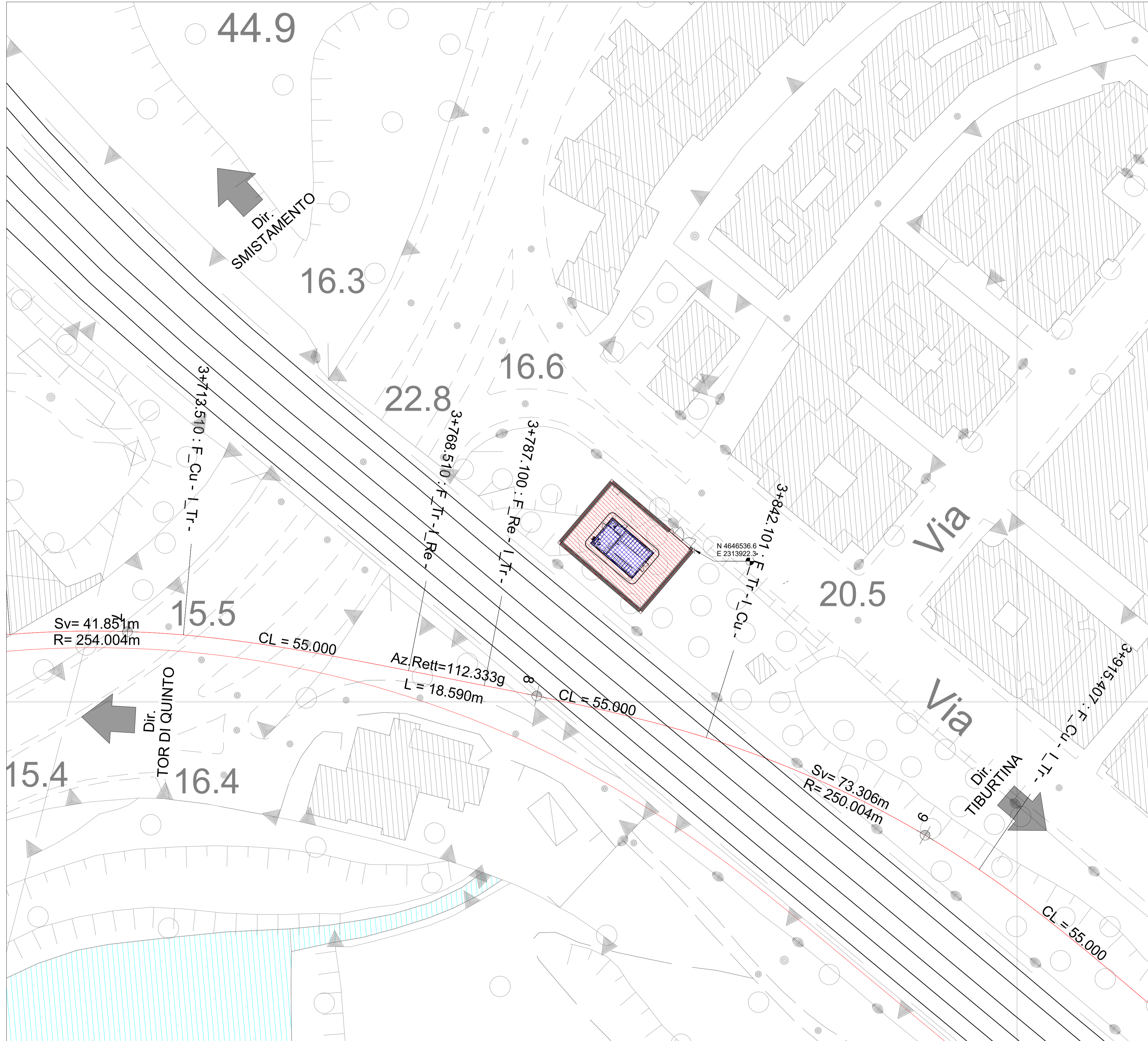
1 Ubicazione Impianto 1 : 500
