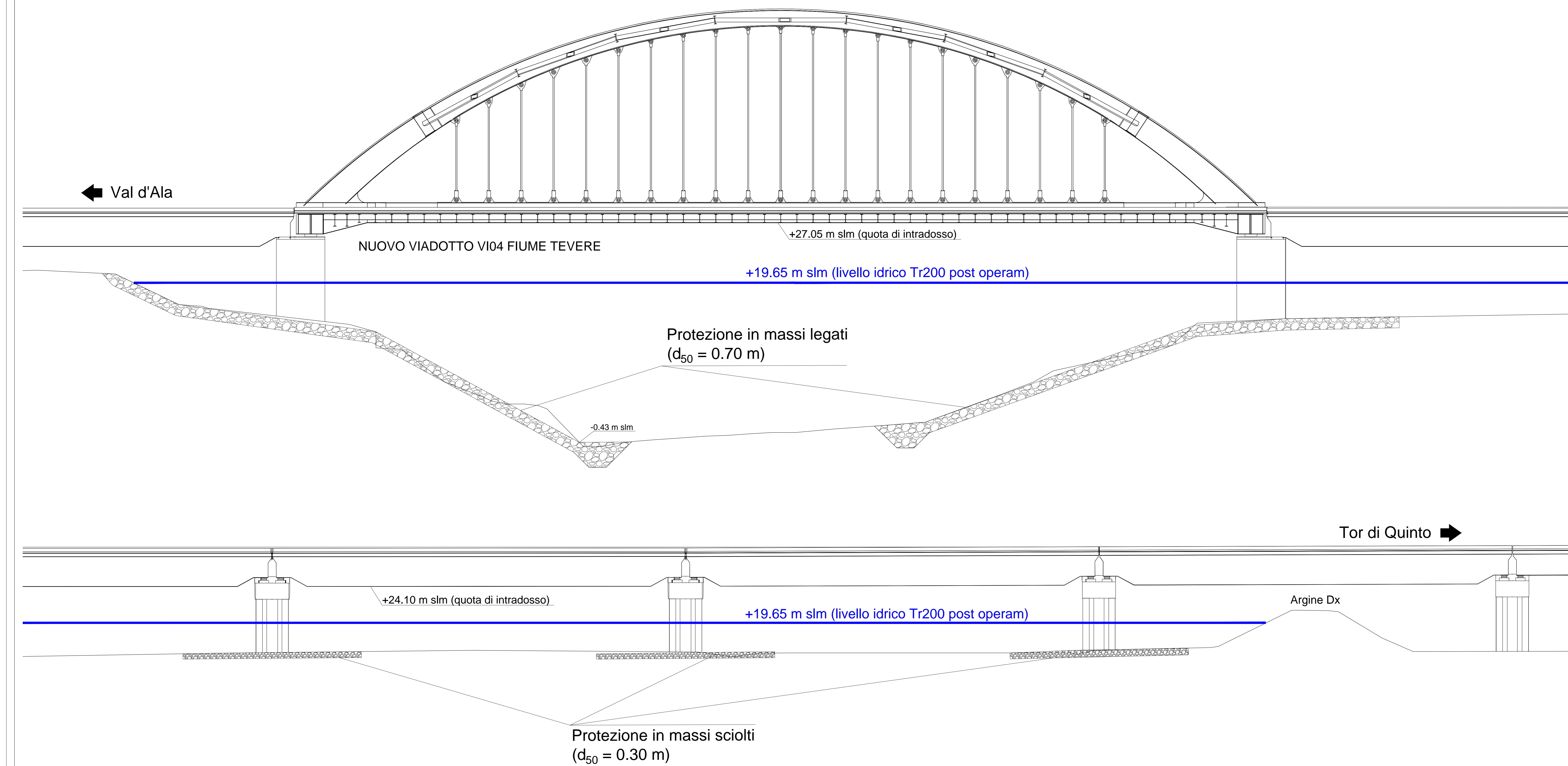
Sezioni sistemazione idraulica - Fiume Tevere - scala 1:200
