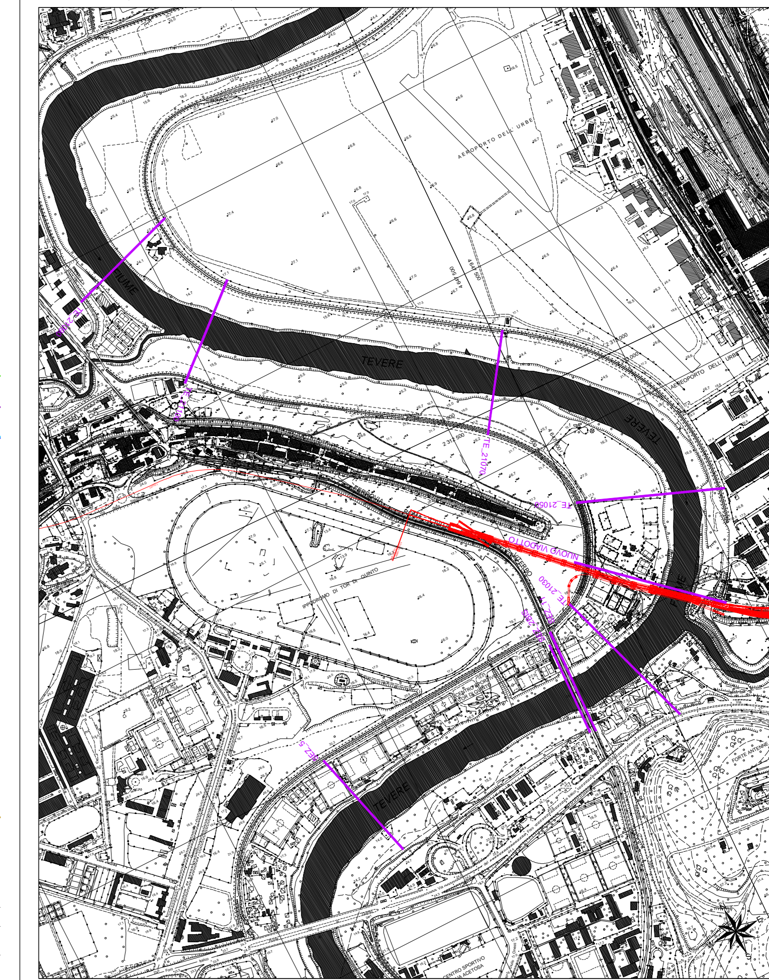
Planimetria (scala 1:10000)
