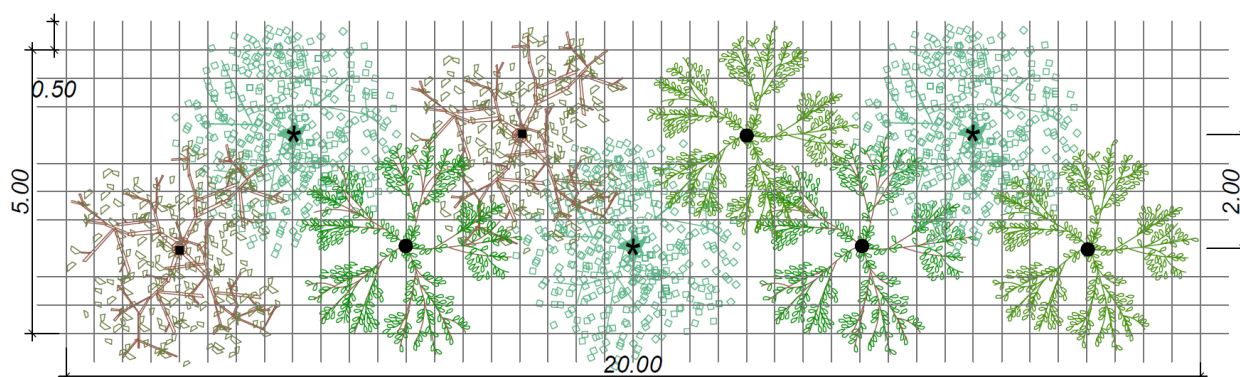
Figura 3-1 Impianto IAAB
