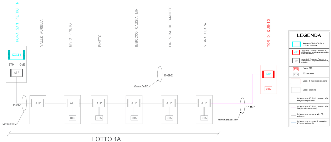
Figura 2: Architettura della rete di trasporto MPLS-TP
